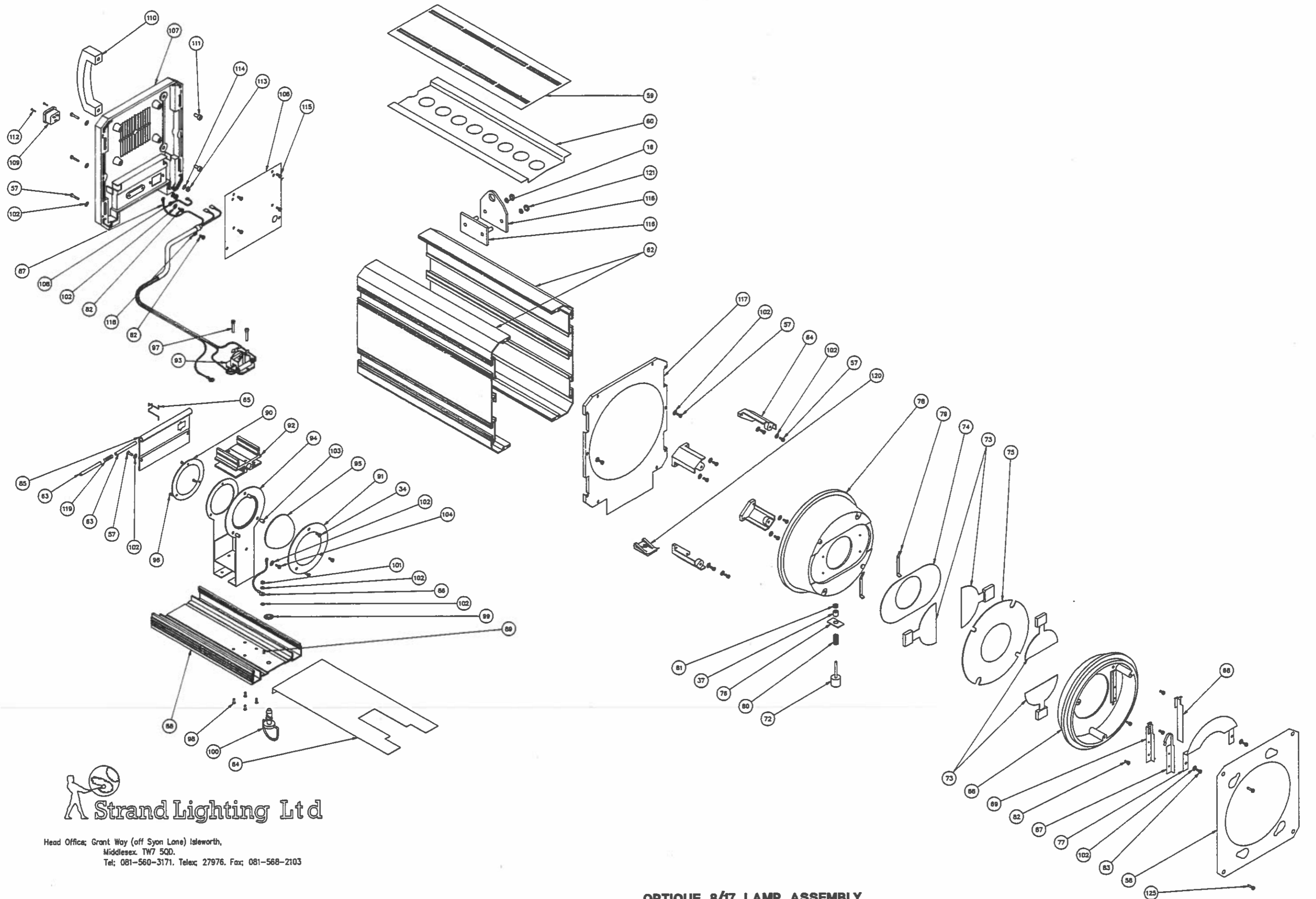
OPTIQUE 8/17 LAMP ASSEMBLY
