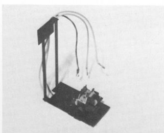
27 499 17 : Lampholder Drop Assby. 27 279 03 : Cable Clip (for above) pkt. 10
