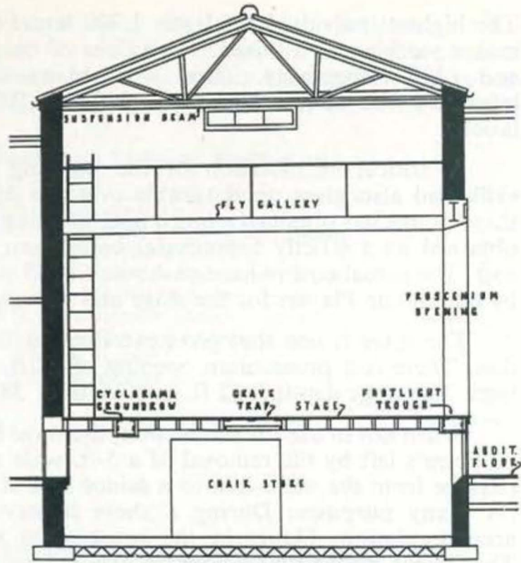
LONGITUDINAL SECTION
