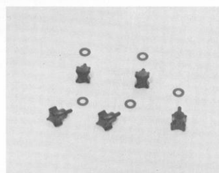
27 210 07 : Lens/Lampray Knob, pkt. 5
